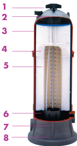
Filtre découpé Star Clear Plus
